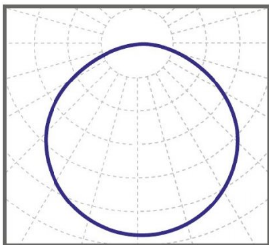
косинусная КСС 115°
